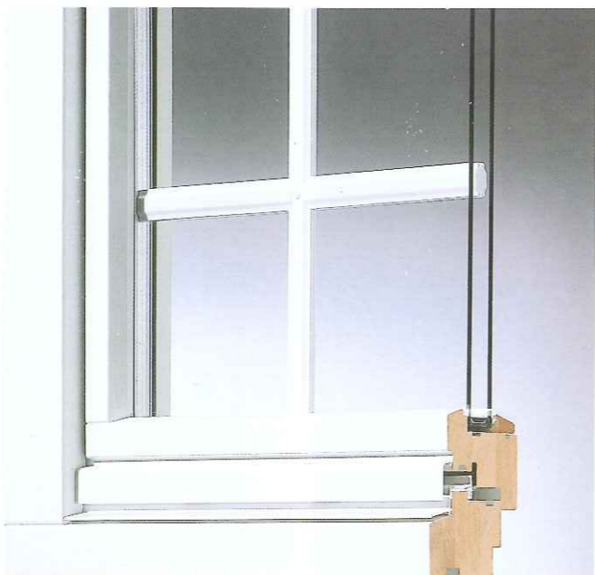
SSR: Sprosse im Scheibenzwischenraum
