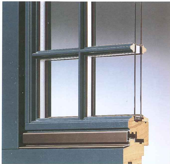
ASA/ZF: Aufgesetzte Zierfalzsporse mit Abstandhaltern
