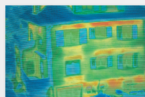
Aufnahme mit rekord Wärmeschutzverglasung (geringer Energieverlust)
